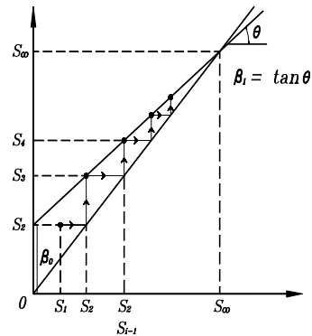
그림 5. 최종침하량 산정(Asaoka)
