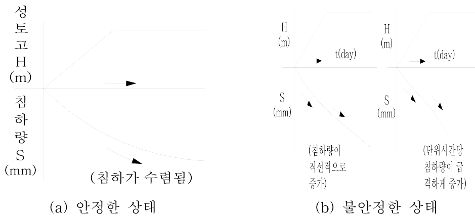
그림 6. 침하량 경시변화
