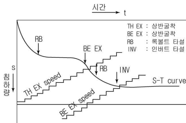
그림 6. 침하량의 경과시간 및 막장진행과의 관계
