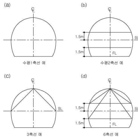
그림 2. 내공변위 및 천단침하 측정의 축선배치(복선터널의 경우)
