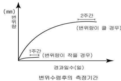
그림 5. 내공변위 구렴후의 측정기간
