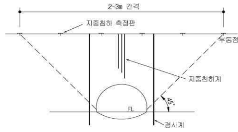
그림 3. 지표침하 및 지중침하 측정의 측정배치 예
