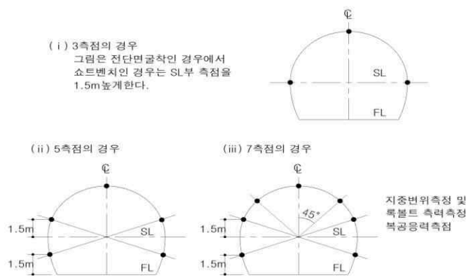
그림 4. 정밀계측의 계측기 배치 (복선단면인 경우)
