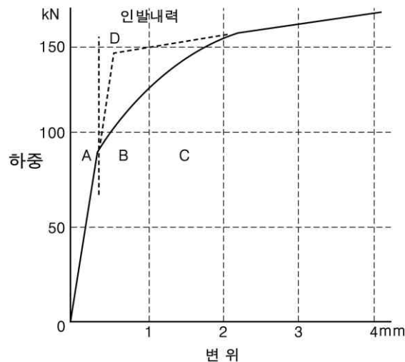
그림 7. 인발시험의 하중-변위곡선
