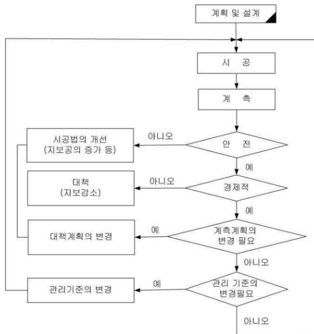
그림 9. 계측결과를 시공관리에 활용하는 순서
